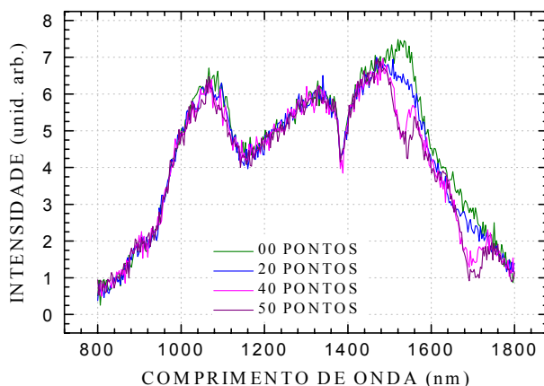
Figura 2: Espectros de transmissão da fibra durante o processo de gravação.
